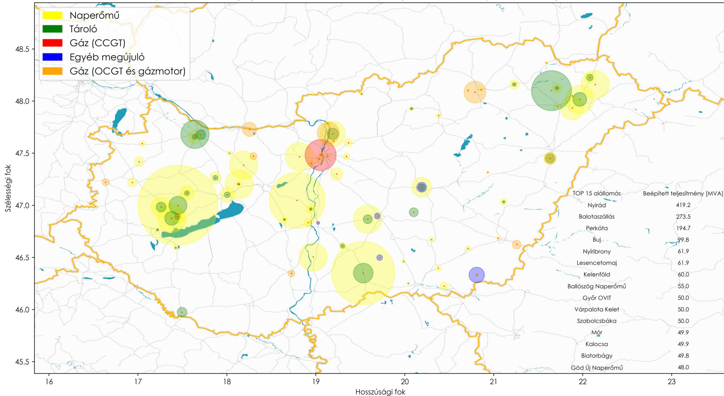
Első közzétételi eljárás keretében végleges MGT-eket és MT felhívást kapott igények beépített teljesítménye energiahordozónkénti bontásban
