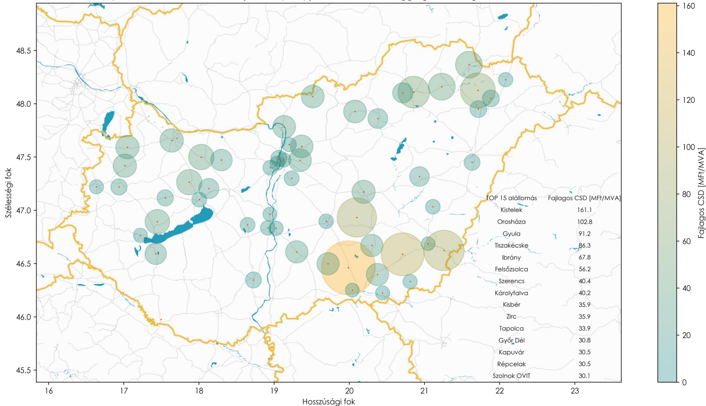
Középfeszültségű hálózatra csatlakozó igények fajlagos közvetett csatlakozási díja a betáplálásra rendelkezésre álló teljesítmény alapján, alállomásokra aggregálva; Átlagos CSD: 27.5 Mft/MVA
