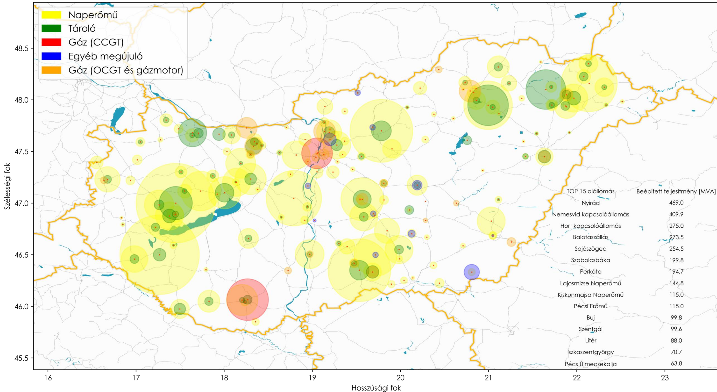
Első közzétételi eljárás keretében jelentkezett igények beépített teljesítménye energiahordozónkénti bontásban
