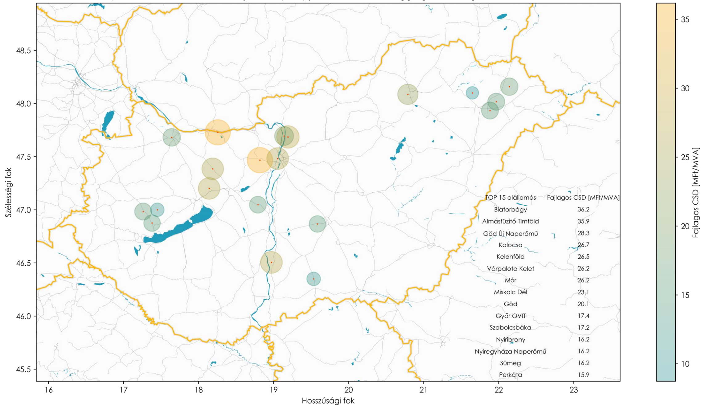
Nagyfeszültségű hálózatra csatlakozó igények fajlagos közvetett csatlakozási díja a betáplálásra rendelkezésre álló teljesítmény alapján, alállomásokra aggregálva; Átlagos CSD: 20.4 MFt/MVA
